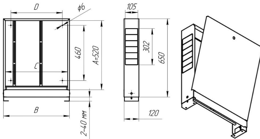
Рис. 1. Шкаф распределительный ШРН «Балтика»
