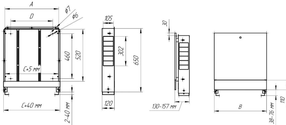
Рис. 2. Шкаф распределительный ШРВ «Балтика»
